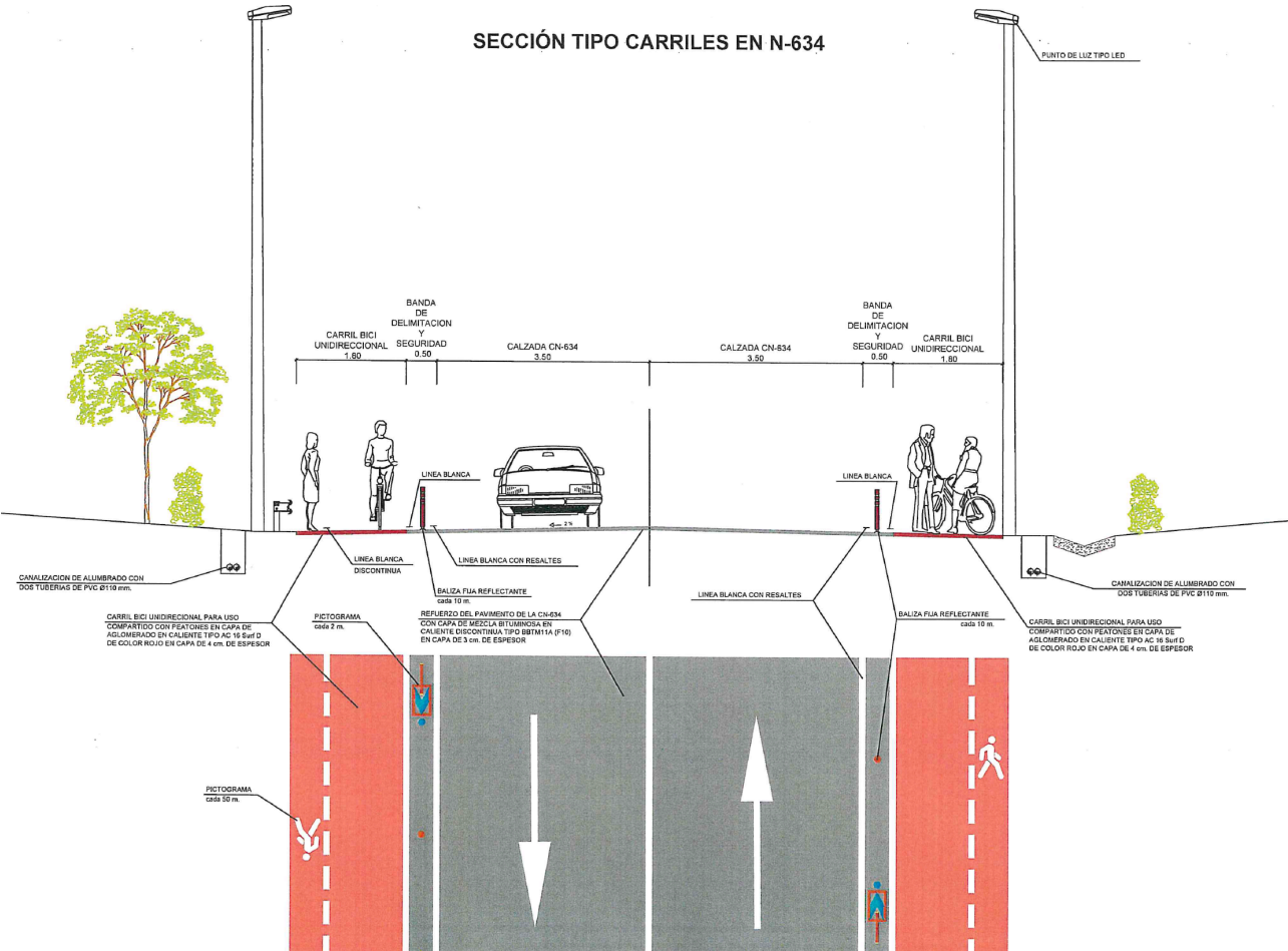
Imagen 58. Movilidad Peatonal. Sección tipo de itinerario peatonal y ciclista por N-634.
