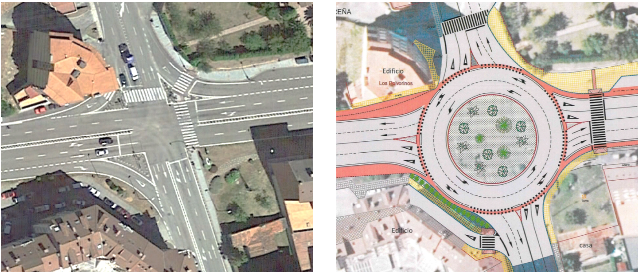
Imagen 59. Carril Bici. Intersección actual (izq.) y glorieta propuesta (dcha.).
