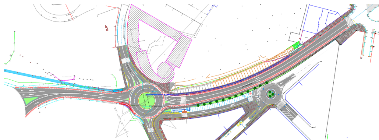
Imagen 62. Carril Bici. C/ Alcalde Parrondo (tramo en La Isla; Proyecto nueva glorieta).
