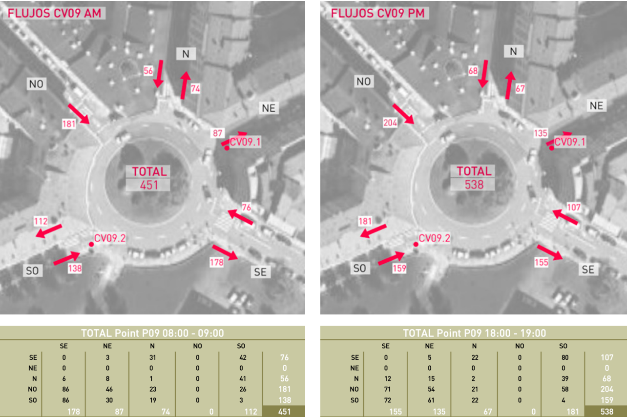
Imagen 35. Punto 9: Glorieta en la Plaza Manuel Llaneza
