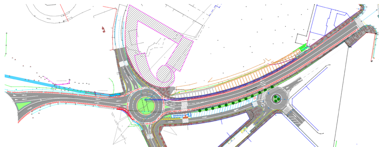
Imagen 71. Proyecto de glorieta en la N-634 (C/ Alcalde Parrondo).
