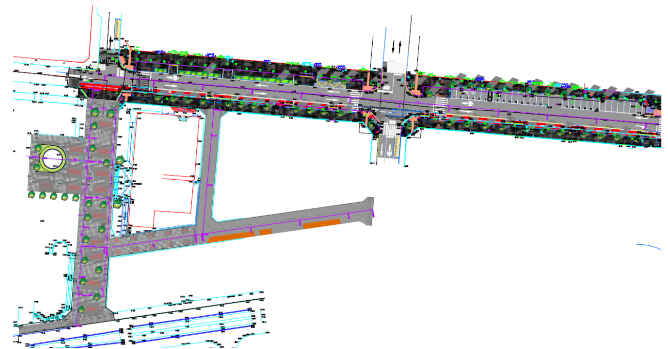
Imagen 56. Movilidad Peonat. Urbanización de la C/ Florencio Rodríguez
