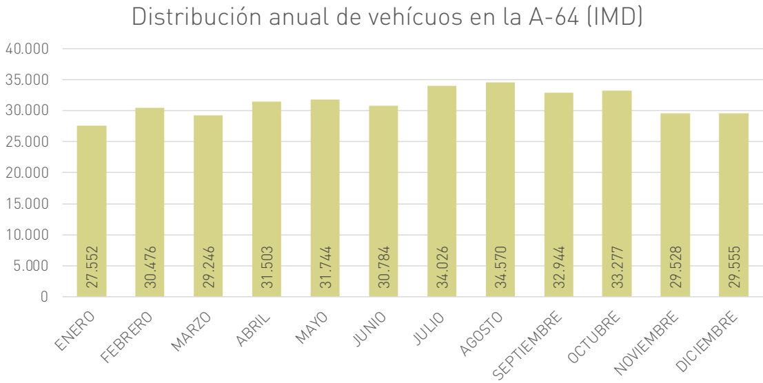
Imagen 24. Distribución anual de vehículos A-64, estación O-7-1.
