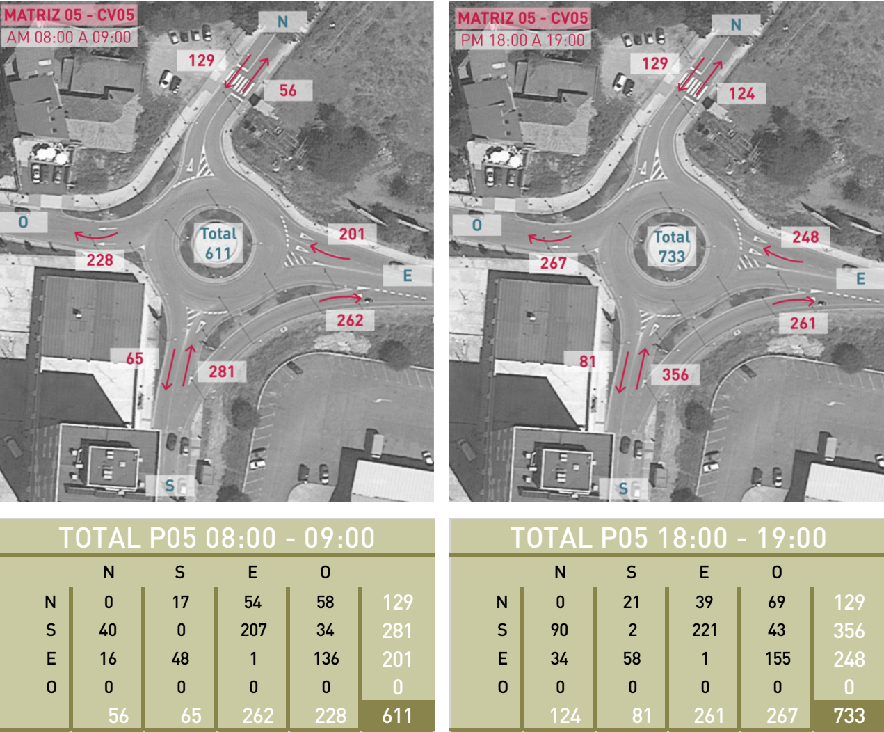
Imagen 31. Punto 5: Glorieta de acceso a Pola de Siero este, unión carretera N-634 y AS-331
