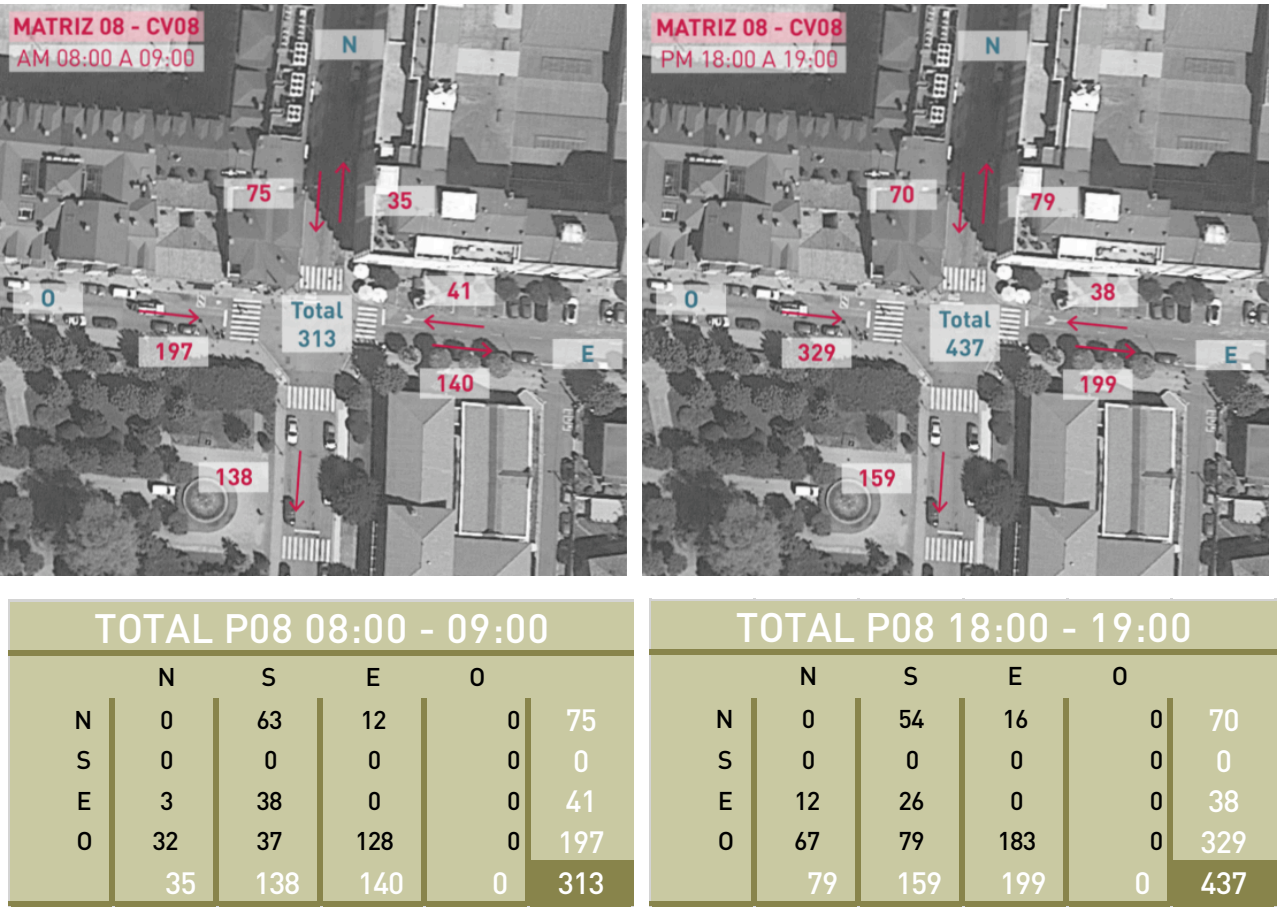
Imagen 34. Punto 8: Intersección entre la carretera AS-377 y Hermanos Felgueroso
