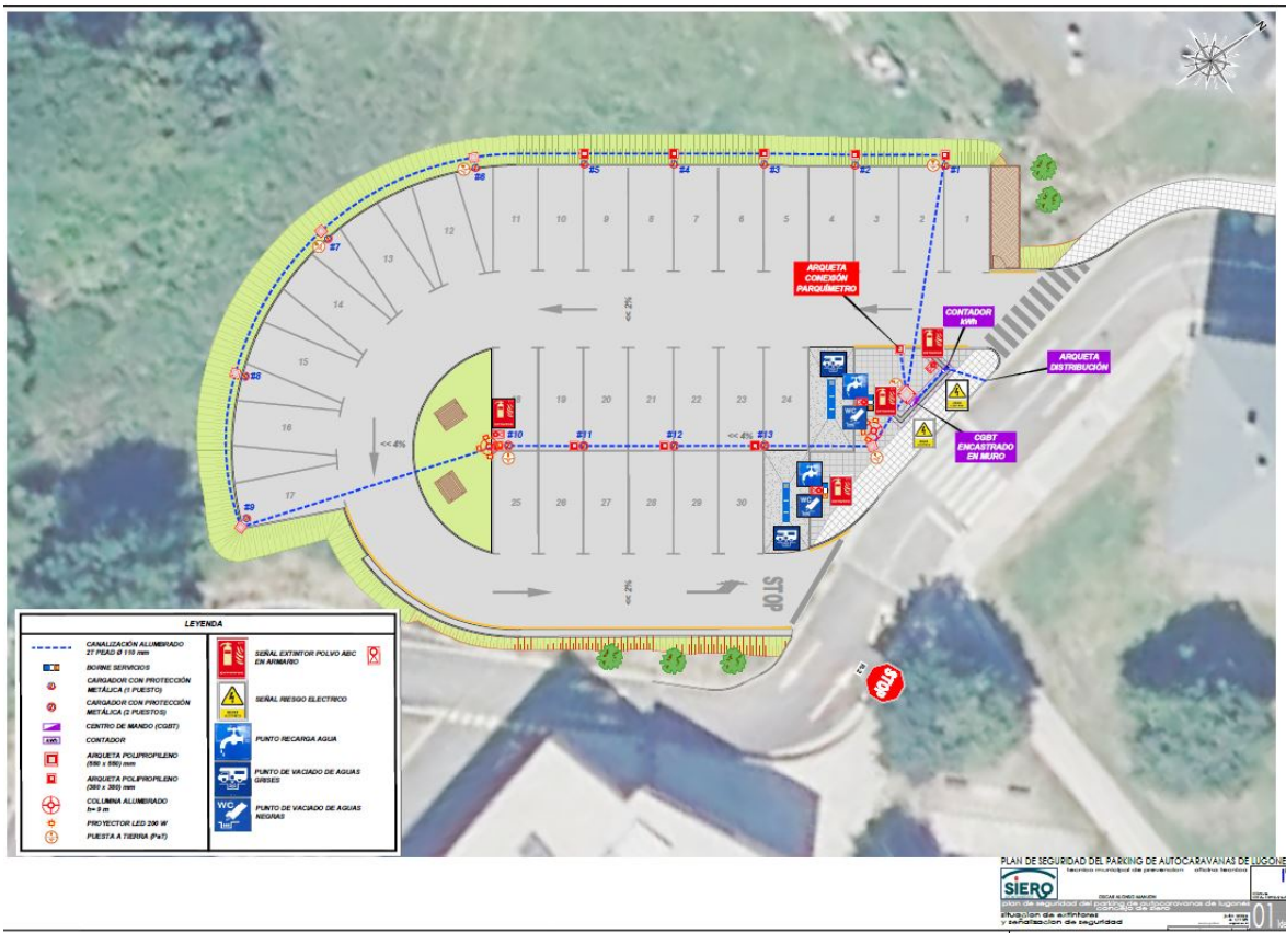
PLANO SITUACIÓN EXTINTORES E INSTALACIONES
