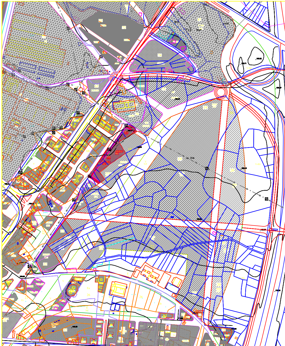
PLANO DE SITUACION SEGUN PLAN GENERAL MUNICIPAL DE ORDENACION DEL CONCEJO DE SIERO
