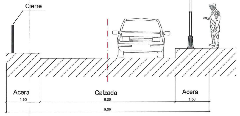
SECCION TIPO VIALES Nº3 - Nº4
