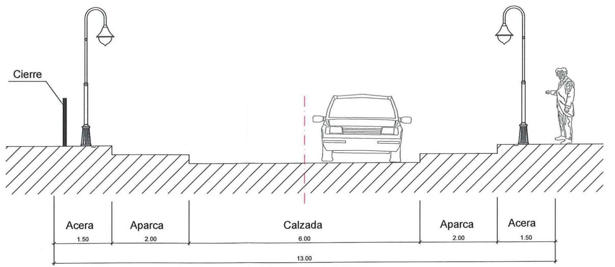
SECCION TIPO VIAL Nº1
