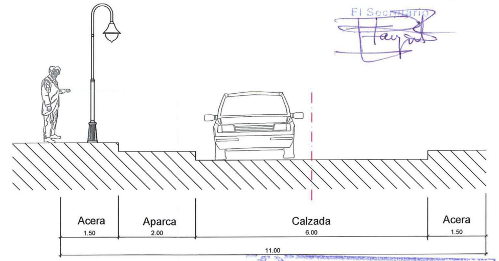
SECCION TIPO VIAL Nº2
